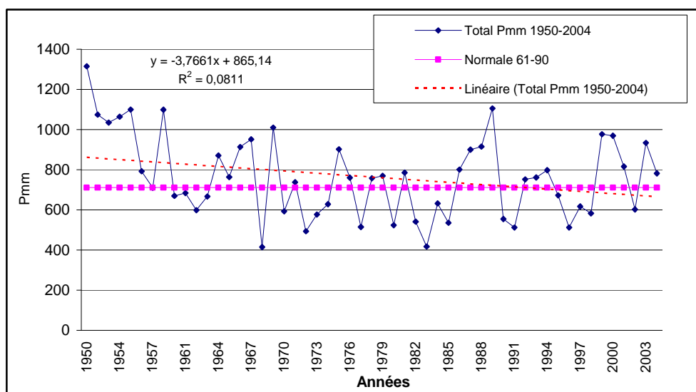
Figure 27 : Variabilité interannuelle de la pluviométrie à Niore du Rip (1950-2004)
